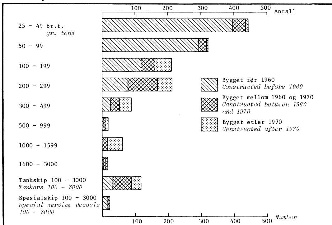
Figur 2. Tallet på skip 1) i leie- og egentransport, etter størrelse/skipstype. 1975 Number of vessels 1) in transport for hire or reward and on own account, by size/type of vessel. 1975
