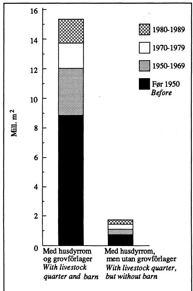
Figur 3.2. Grunnflate av driftsbygningar med husdyrrom, etter byggjeår. 1 Heile landet. 1989. Mill. m 2 Ground area of farm buildings with livestock quarter, by year of construction. 1 The whole country. 1989. Mill. m 2
