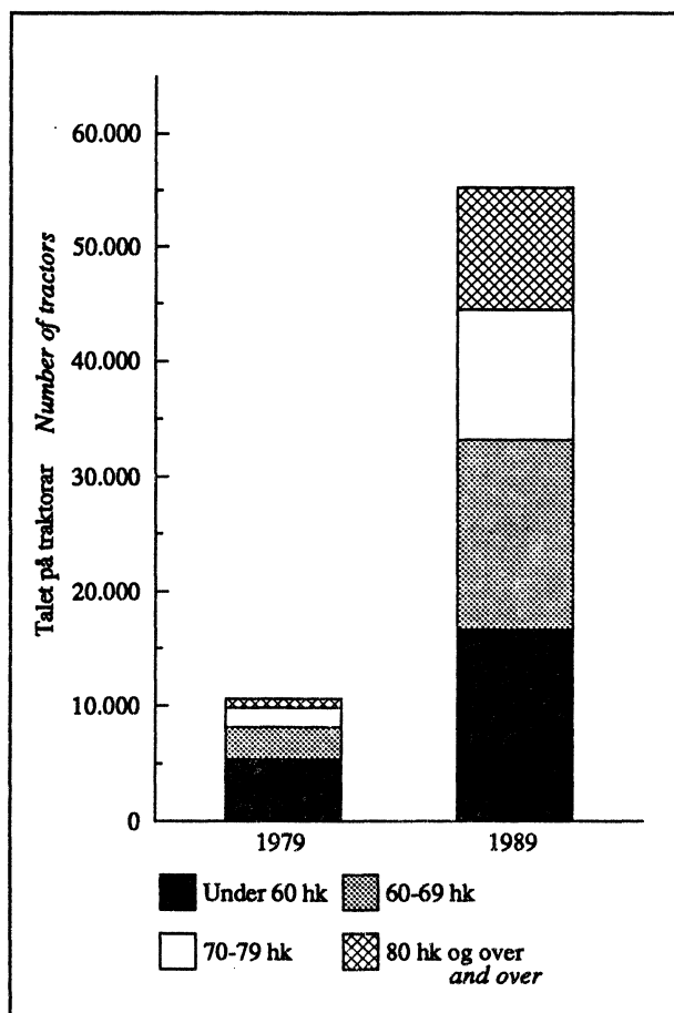
Figur 2.3. Talet på 4-hjuls traktorar med 4-hjuls drift, etter motorstyrke. 1 Heile landet. 1979 og 1989 Number of 4-wheeled tractors with 4-wheel drive, by engine power. 1 The whole country. 1979 and 1989
