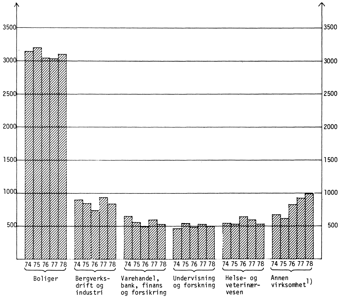
Bygg under arbeid pr. 30. juni 1974-1978. Golvflate i 1 000 m 2
