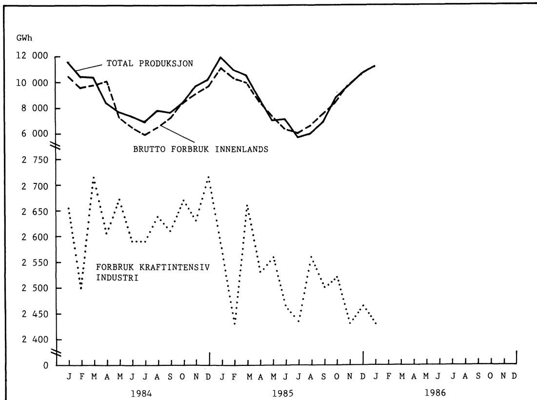
Figur 2. Produksjon, bruttoforbruk, forbruk i kraftintensiv industri. Måned
