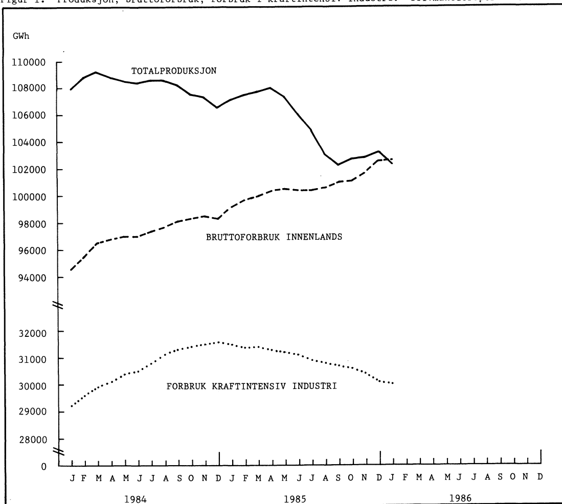
Figur 1. Produksjon, bruttoforbruk, forbruk i kraftintensiv industri. Tolvmånedersperioder
