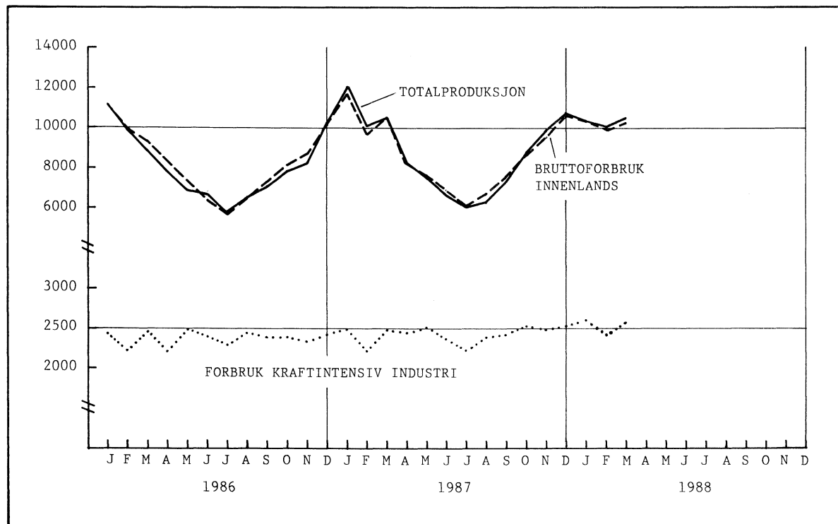
Figur 2. Produksjon, bruttoforbruk, forbruk i kraftintensiv industri. Måned
