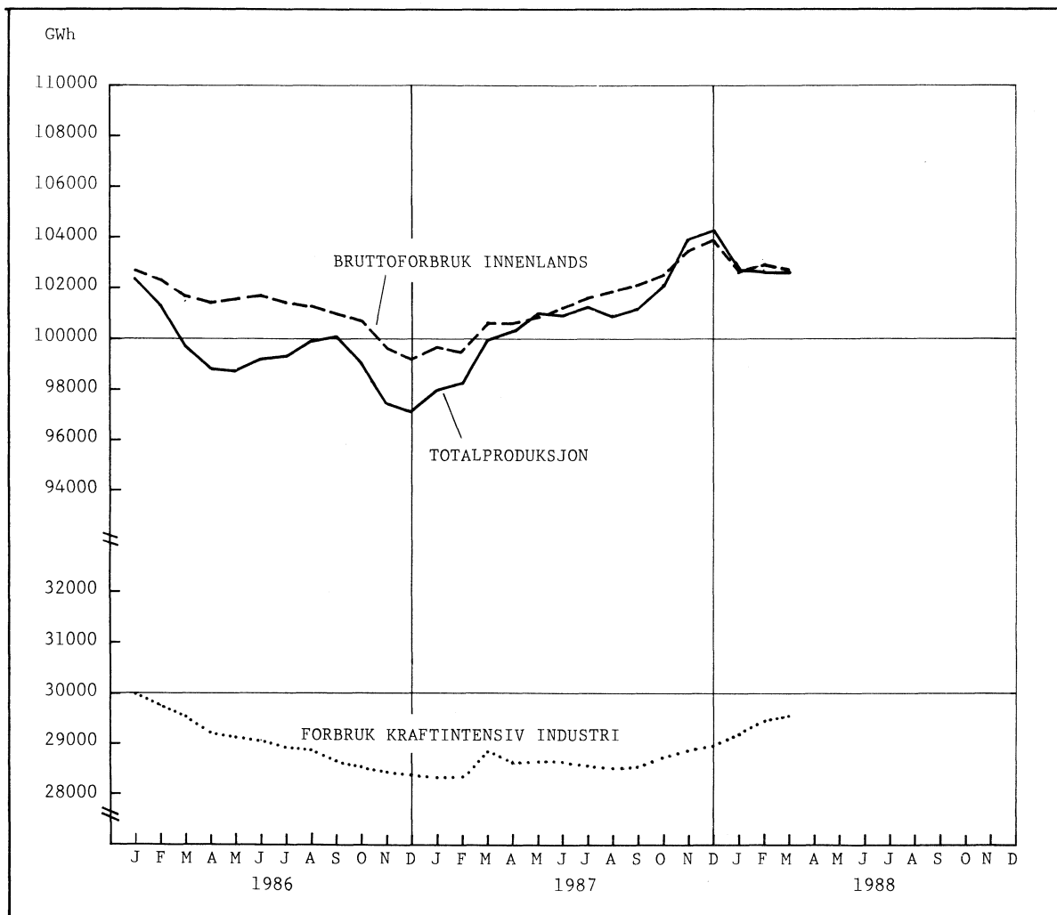
Figur 1. Produksjon, bruttoforbruk, forbruk i kraftintensiv industri. Tolv månedersperioder
