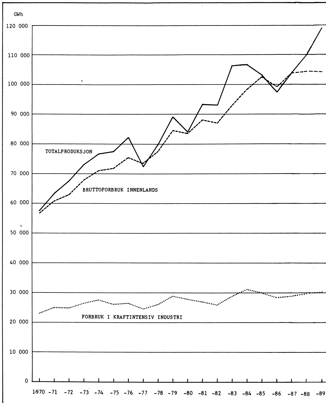
Figur 3. Produksjon, bruttoforbruk, forbruk i kraftintensiv industri. 1970-1989
