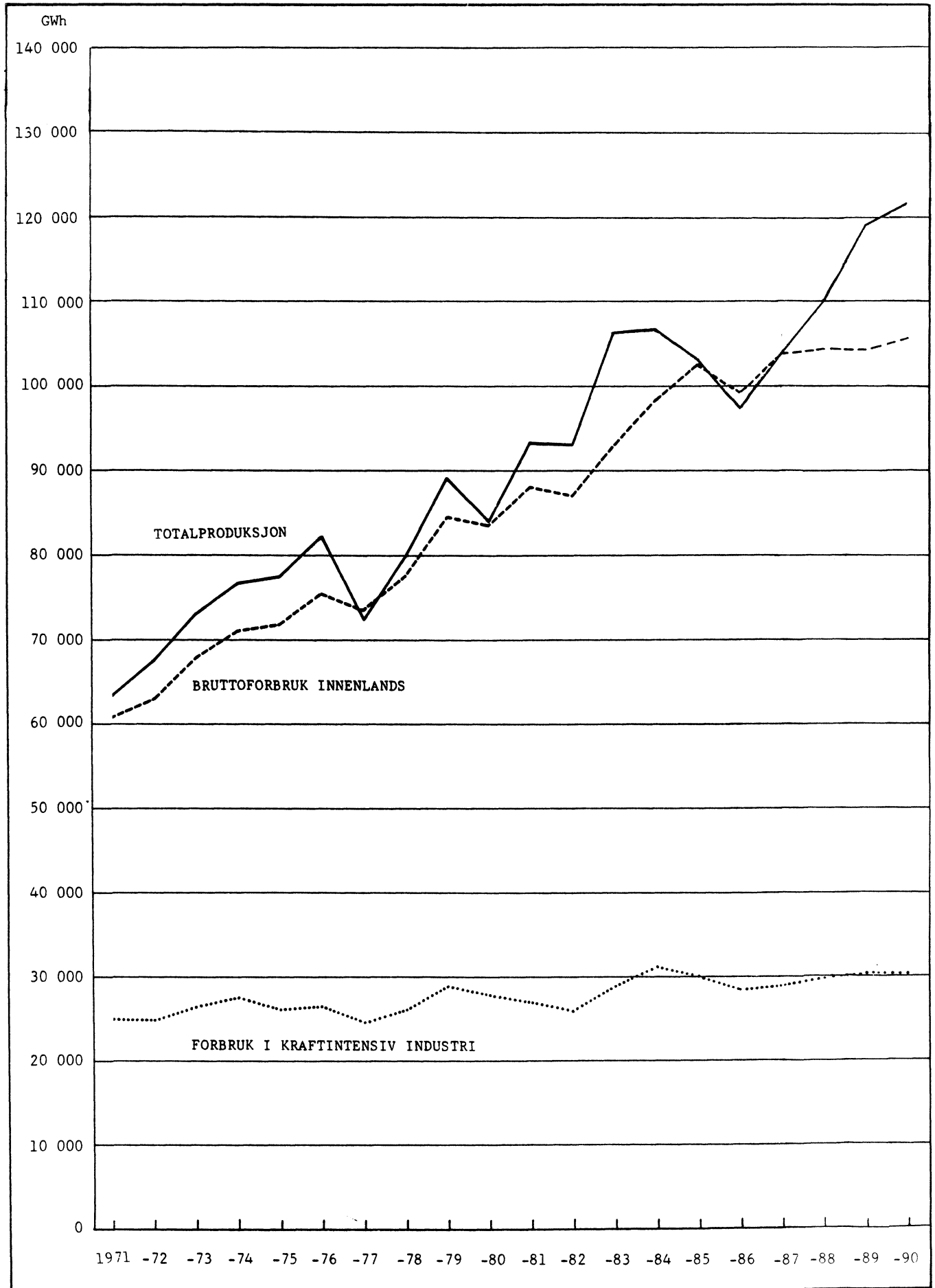
Figur 3. Produksjon, bruttoforbruk, forbruk i kraftintensiv industri. 1971-1990
