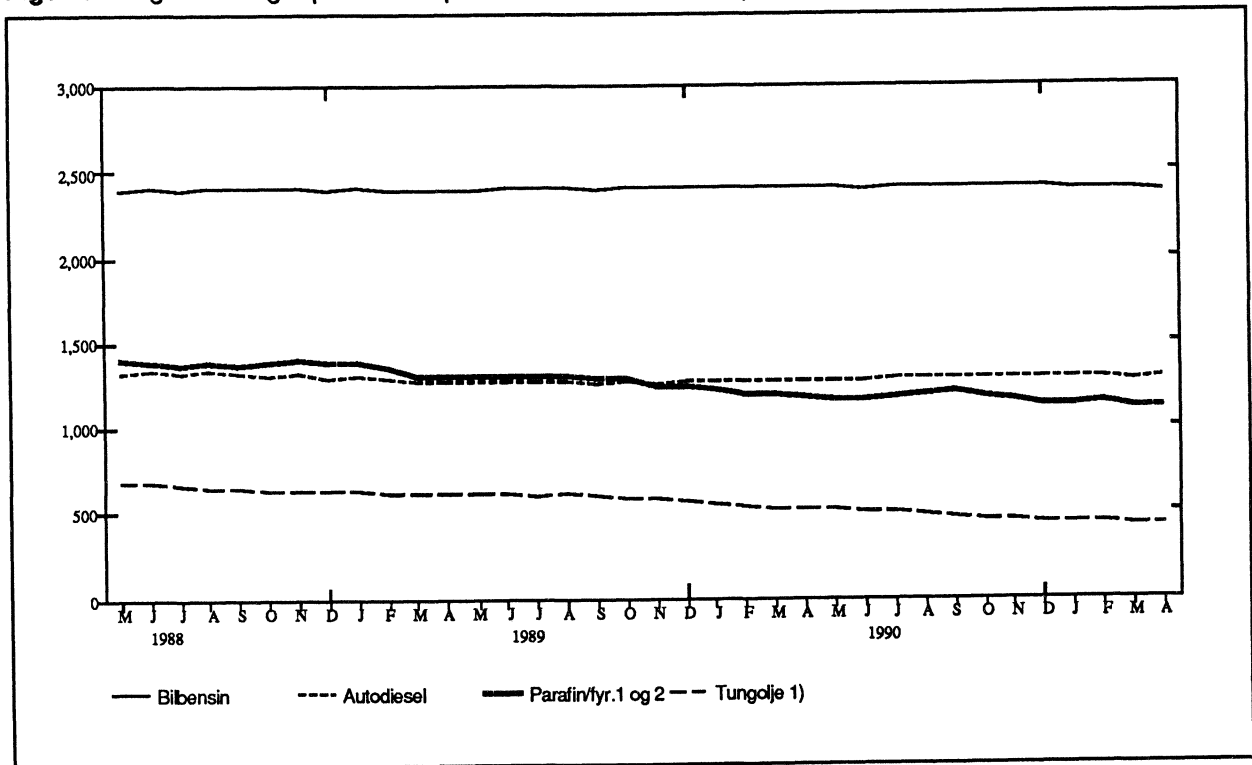
Figur 3. Salg av utvalgte petroleumsprodukter. Tolvmånedersperioder. Mai 1988 - april 1991. Mill. liter
