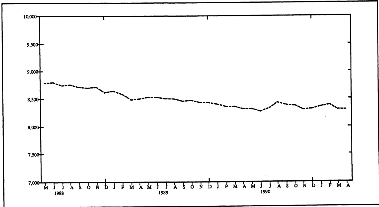
Figur 2. Salg av petroleumsprodukter i alt. Tolvmånedersperioder. Mai 1988 - april 1991. Mill. liter
