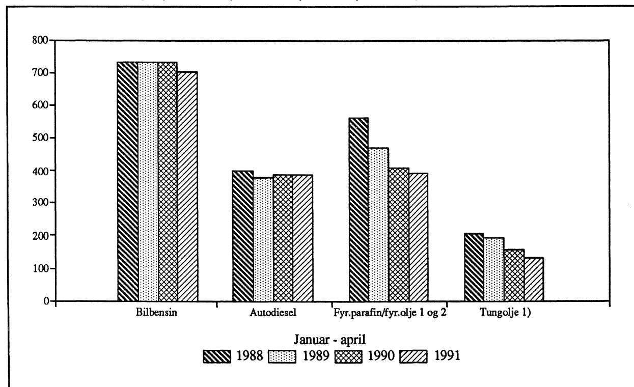
Figur 1. Salg av utvalgte petroleumsprodukter i perioden januar - april. 1988 - 1991. Mill. liter
