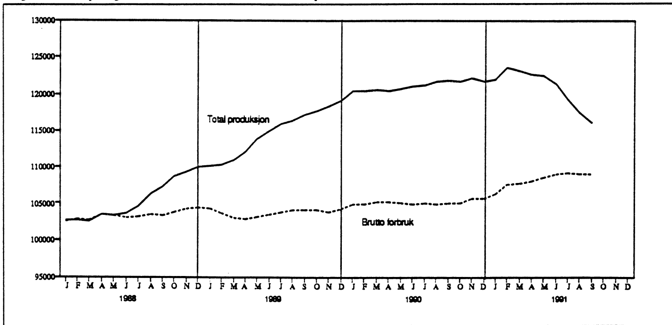
Figur 3. Produksjon og forbruk av elektrisk kraft. Tolv månedersperioder. GWh
