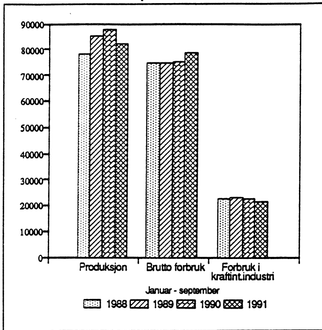
Figur 2. Produksjon, brutto forbruk og forbruk i kraftintensiv industri. Januar-september. GWh
