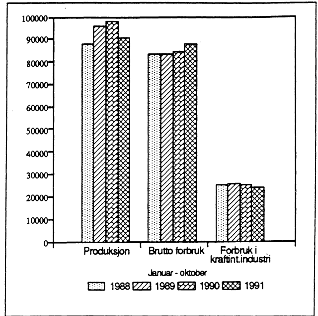
Figur 2. Produksjon, brutto forbruk og forbruk i kraftintensiv industri. Januar-oktober. GWh
