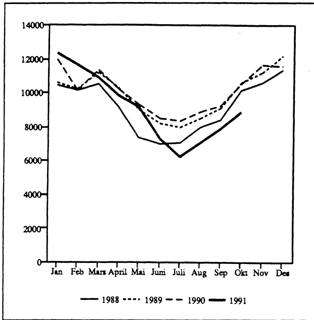
Figur 1. Produksjon av elektrisk kraft. Måned. GWh
