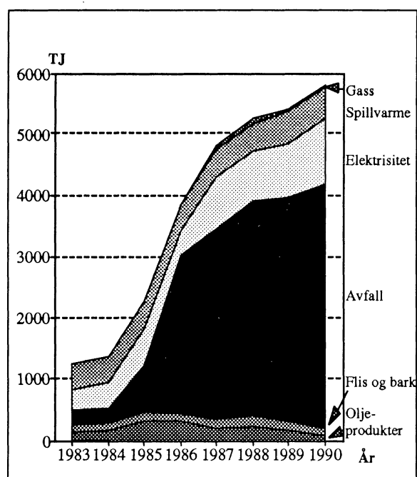
Figur 3. Forbruk av brensel til bruttoproduksjon av fjernvarme. 1983-1990. TJ
