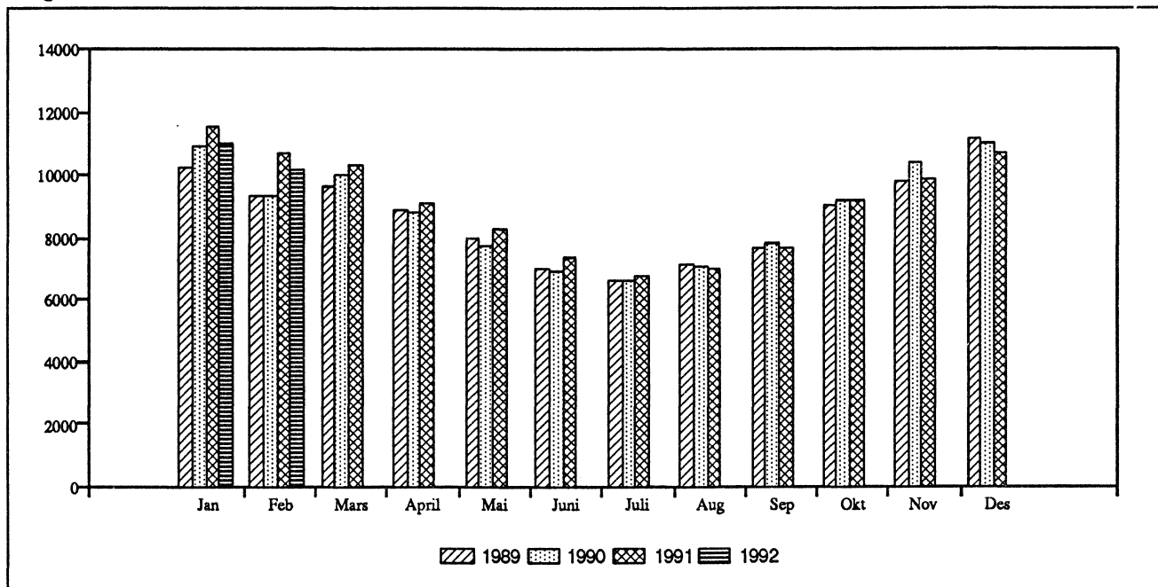
Figur 3. Brutto forbruk av elektrisk kraft. Måned. GWh
