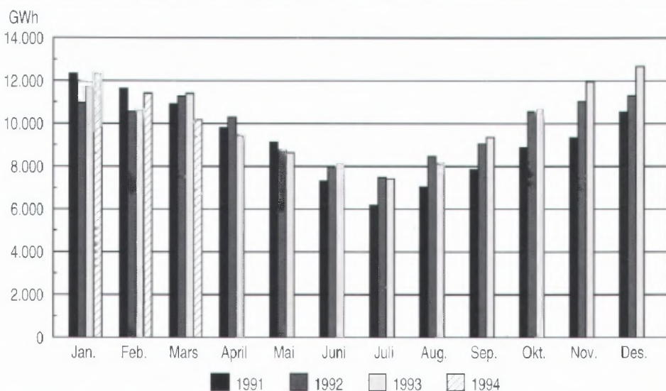
Produksjon av elektrisk kraft. Måned. GWh
