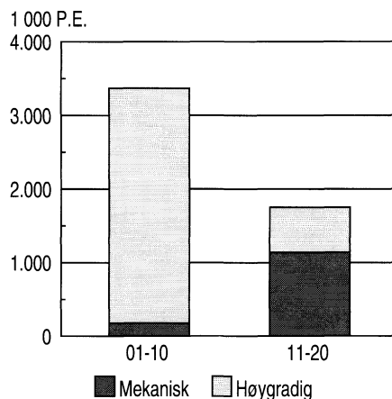
Hydraulisk rensekapasitet i alt for kommunale avløpsrenseanlegg, etter renseprinsipp. Fylke 01-10 og fylke 11-20 1 . 1995. 1 000 P.E.
