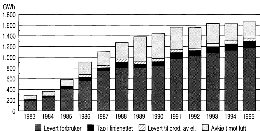
Bruttoproduksjon av fjernvarme. GWh
