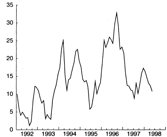
Fig. 7.4 Spotpris elektrisk kraft Øre pr. kWh
