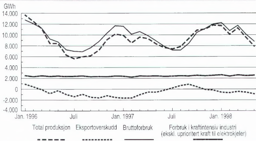
Produksjon, forbruk og eksportoverskudd av elektrisk kraft per måned. Januar 1996-mai 1998. GWh
