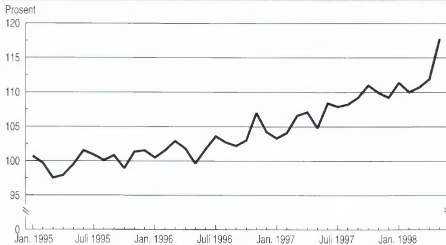
Detaljomsætning eksklusiv motorkjøretøyer og bensin i volum, sesongjustert. Januar 1995-mai 1998. 1995=100
