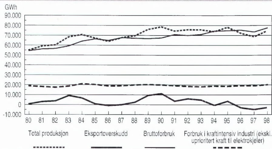
Produksjon, forbruk og eksportoverskudd av elektrisk kraft i januar-august, 1980-1998. GWh
