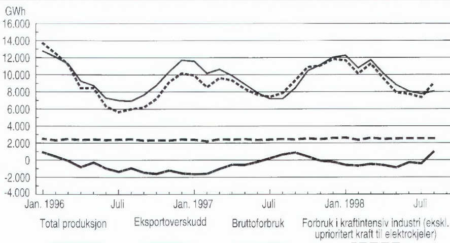
Produksjon, forbruk og eksportoverskudd av elektrisk kraft per måned, Januar 1996-august 1998. GWh
