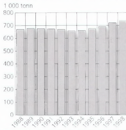
Nyttelastkapasitet for godsbiler med nyttelast 1 tonn og over. 1988-1998. 1 000 tonn
